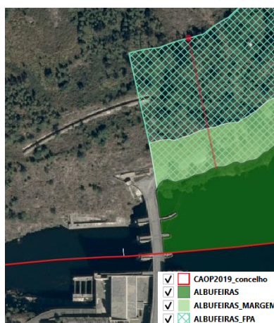
Figura 6 | Exemplo de correta delimitação da FPA, definida a partir da linha limite do leito da albufeira, incluindo a respetiva margem (novas OENR).
