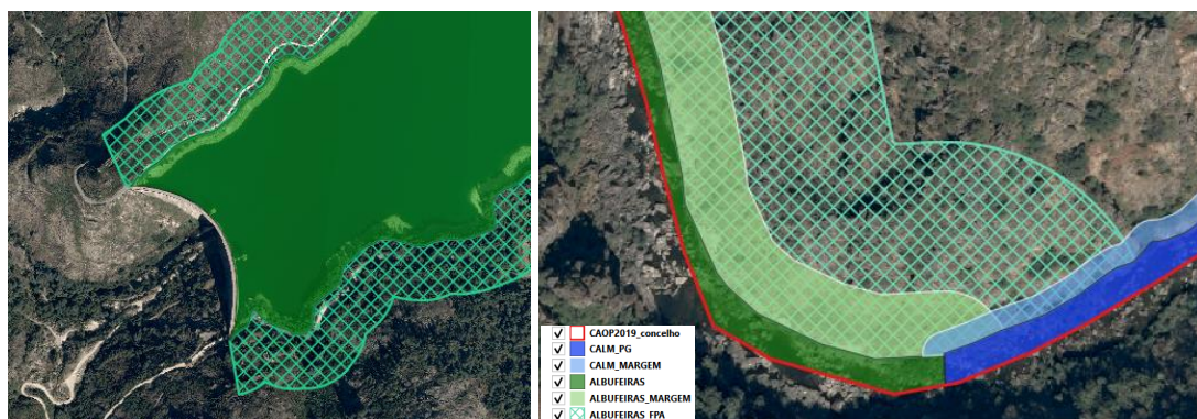
Figuras 7 e 8 | Exemplo de correta delimitação da FPA: Esquerda - corte a jusante da barragem (excluindo a própria estrutura); Direita - interrupção no limite do leito do curso de água poligonal, eliminando tal sobreposição.
