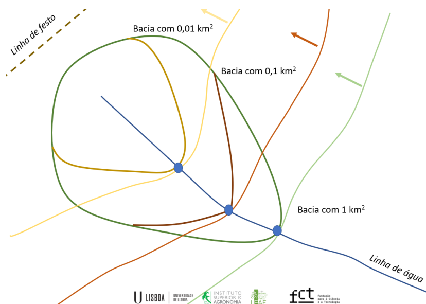
Figura 7 – Esquema de delimitação das cabeceiras e da variação do início da rede hidrográfica em função da área de drenagem
