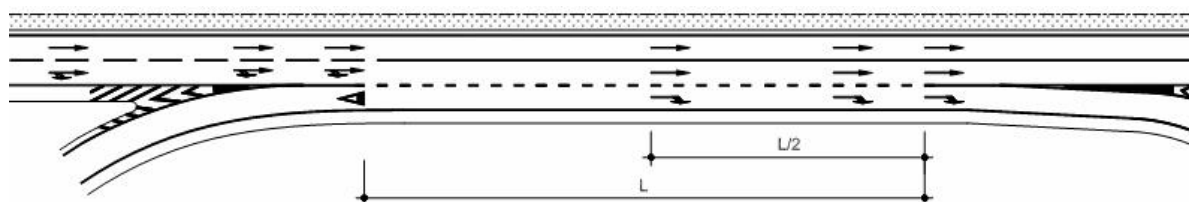
Figura 17 - Setas de selecção em via de entrecruzamento
