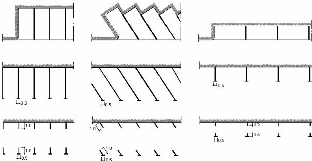
Figura 11 - Marcação de lugares de estacionamento
