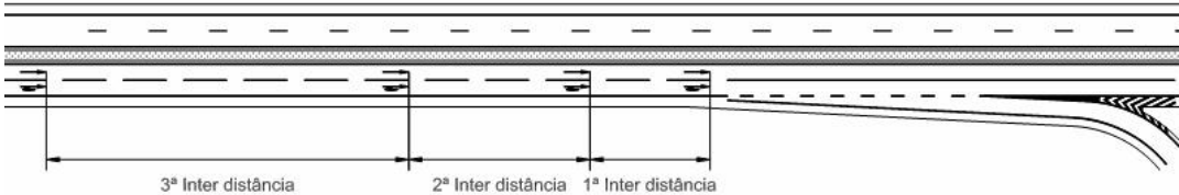
Figura 15 - Setas de selecção em intersecções desniveladas
