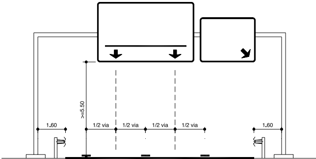
Figura 34 – Exemplos de colocação de sinais grandes dimensões
