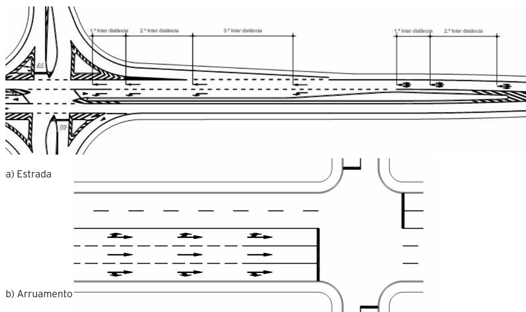
Figura 16 - Setas de selecção em intersecções de nível
