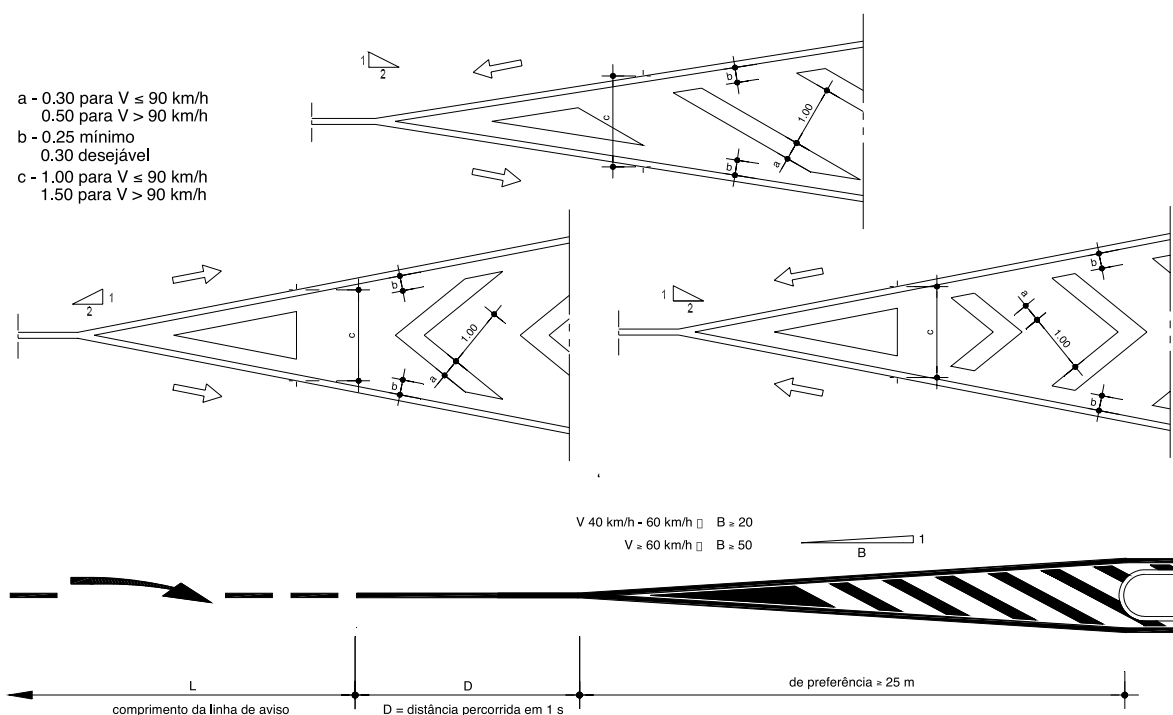
Figura 20 - Características das raia oblíquas
