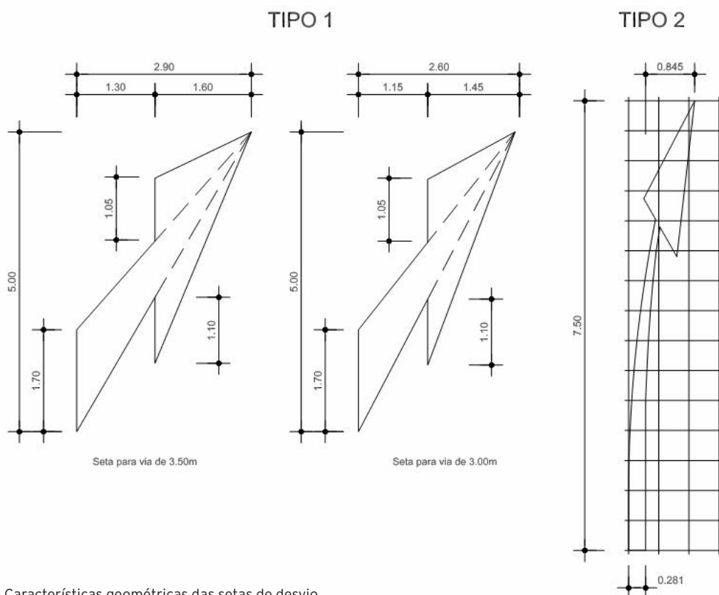
Figura 13 - Características geométricas das setas de desvio
