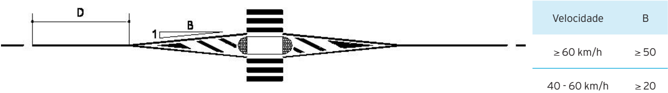
Figura 23 - Raias oblíquas numa travessia com refúgio para peões
