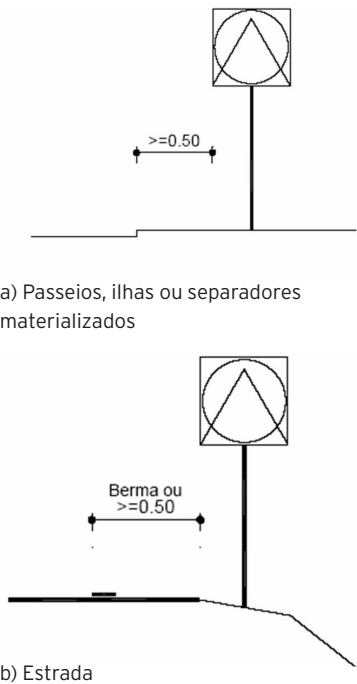
Figura 26 - Colocação transversal dos sinais verticais
