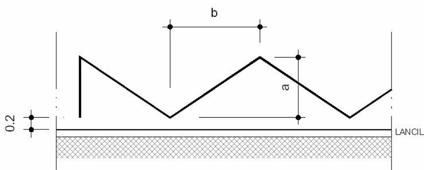
Figura 9 - Linha em ziguezague (M14)
