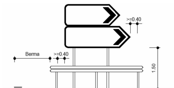
Figura 32 - Exemplos de colocação de sinais de direcção
