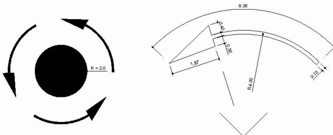
Figura 19 - Exemplo de dimensionamento de setas em mini-rotundas
