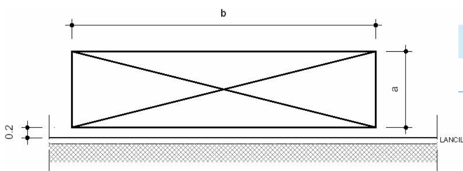
Figura 10 - Marca de paragem e estacionamento para cargas e descargas (M14a)
