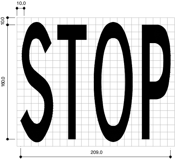
Figura 7 - Inscrição de “STOP”
