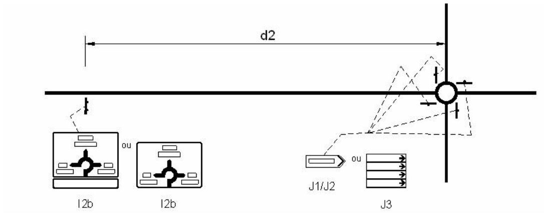
Figura 46 - Rotunda
