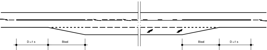
Figura 5 - Via de lentos
