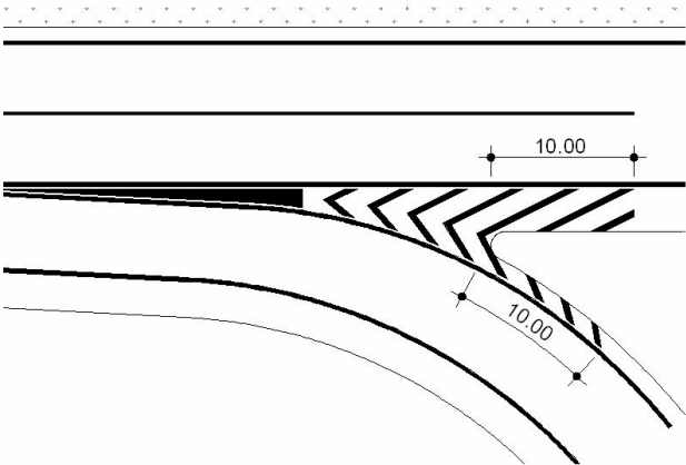
Figura 24 - Raias oblíquas em intersecções desniveladas
