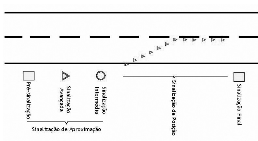
Figura 50 - Esquema de implantação da sinalização temporária
