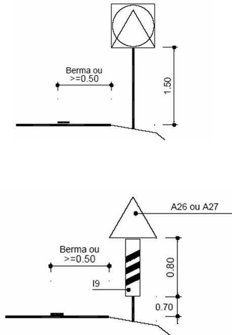
Figura 30 - Exemplos de colocação de sinais de código
