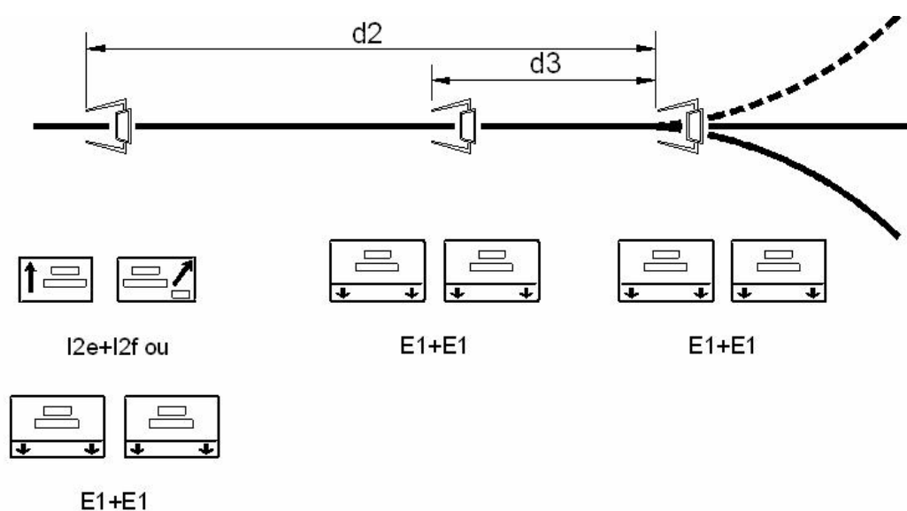
Figura 42 - Separação de duas ou mais vias de tráfego em faixa com quatro ou mais vias de tráfego
